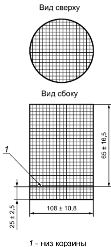
Рисунок 1 - Проволочная корзина
