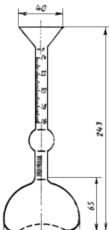
Рисунок 1 - Прибор Ле-Шателье
