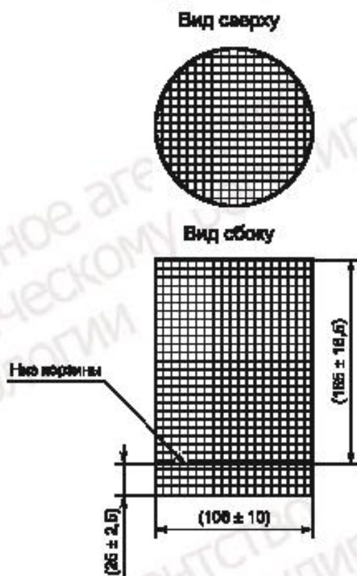
Рисунок 1 — Проволочная корзина
